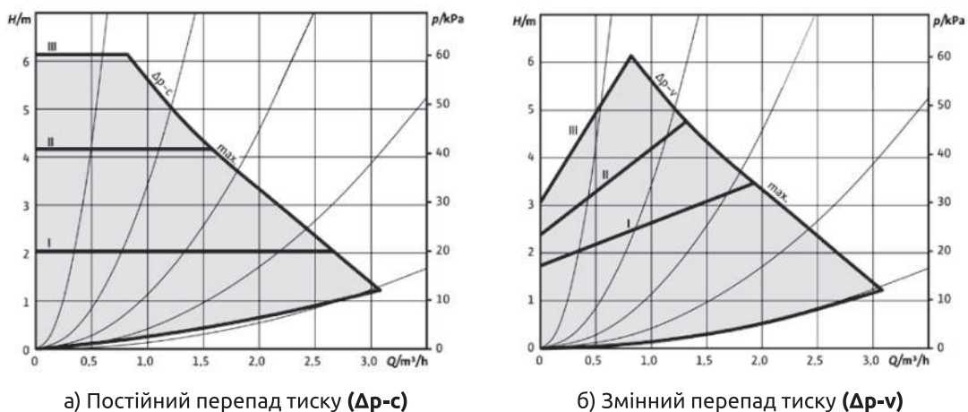
Малюнок 9 – Характеристики насоса Wilo PARA 15-130/6-43/SC для режимів.
