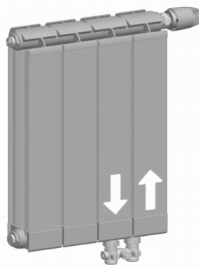
Нижняя связь MV, TV вправо или влево
